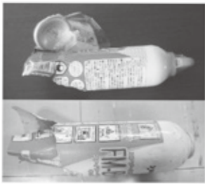
破裂事故を起こしたヤマトプロテック社製 エアゾール式簡易消火具
