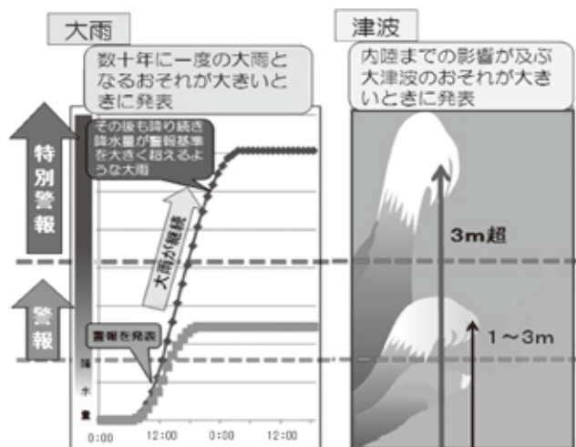
「特別警報」のイメージ図 (気象庁HP「気象等の知識」より引用)
