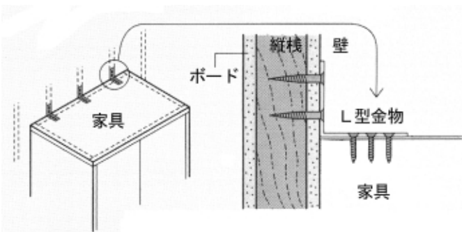
木ネジは最低35mm以上の物を使用してください。
