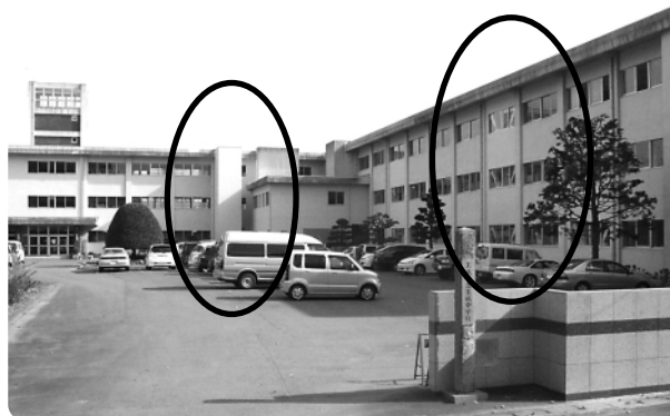
中央の○印はエレベーター、右の○印は鉄骨補強柱が入った壁
